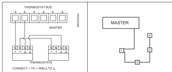
Tilkobling av termostater til Master.
