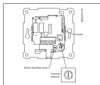
Innstilling av kanal (varmekurs) ved bruk av skruetrekker. Ved trådløs funksjon trykkes knappen under kanalvelgeren inn i ca. 2 sek.
